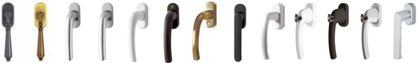
Fer patiné Laiton vieilli F9 Sécustik F9 Blanc Noir Laiton poli A saillie réduite noire Sécustik Blanc Blanc Noir F9 F9 design
