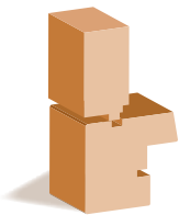
Tapée (intérieure ou extérieure) rapportée pour isolation de 60 à 200 mm
